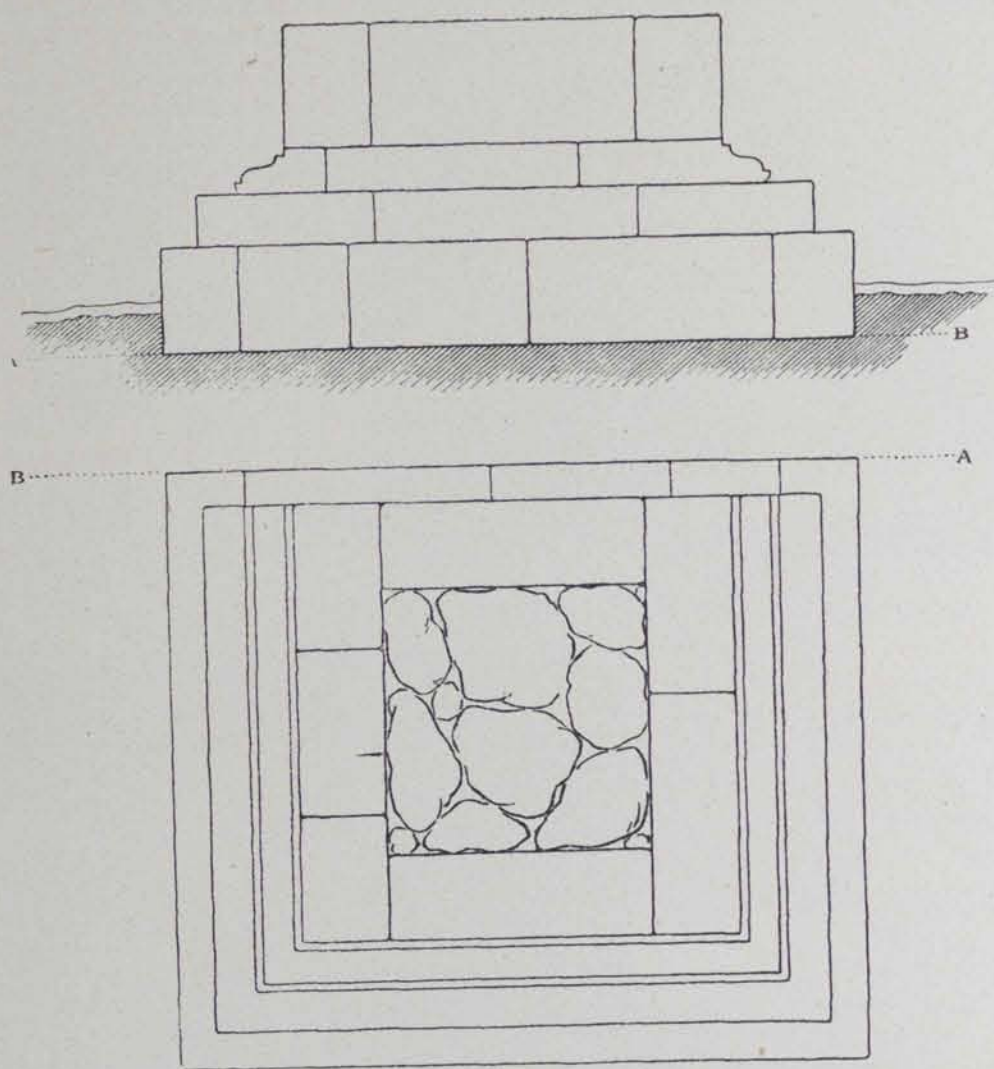
Fig. 201. — Necròpolis de Tarragona. Basament de sepulcre Escala 1 : 50
