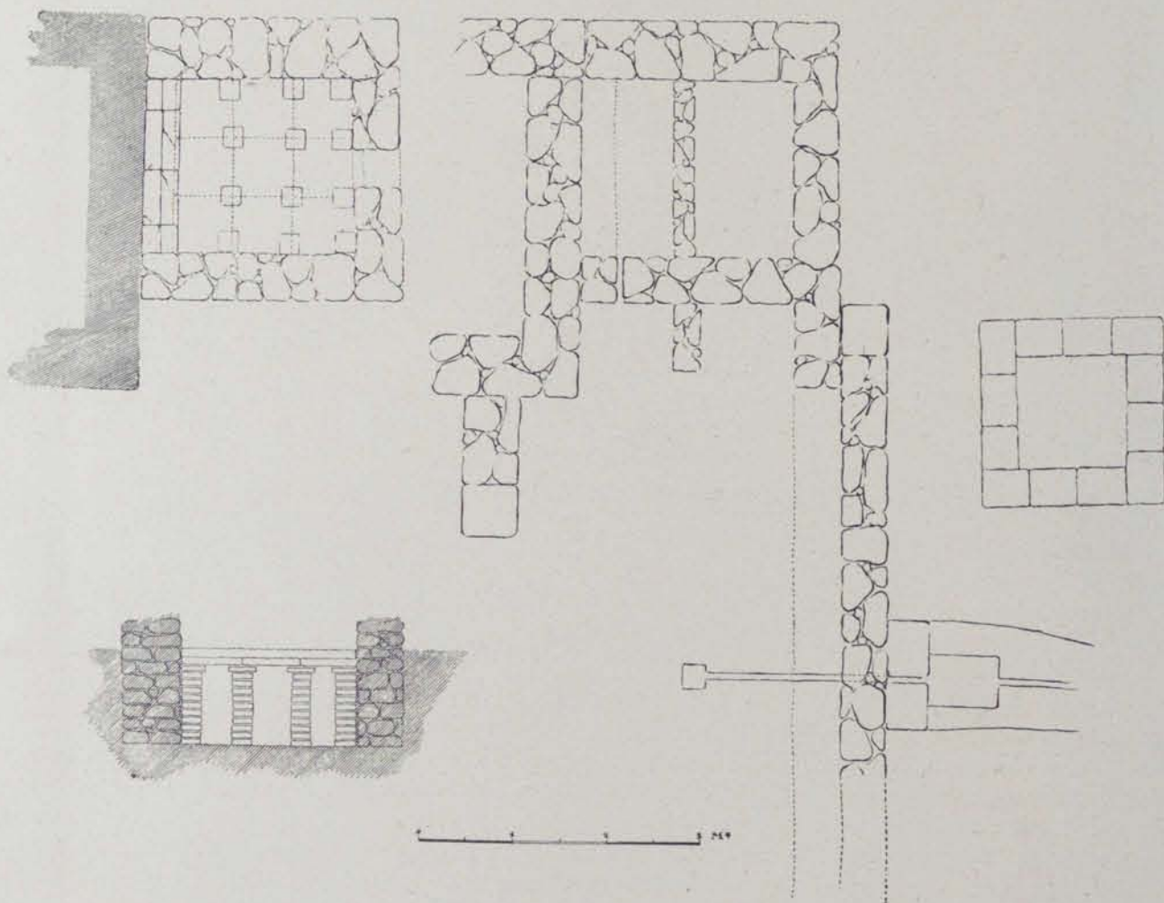
Fig. 196. — Necròpolis de Tarragona. Plan i secció de l'hipocauste (XI del plan general)
